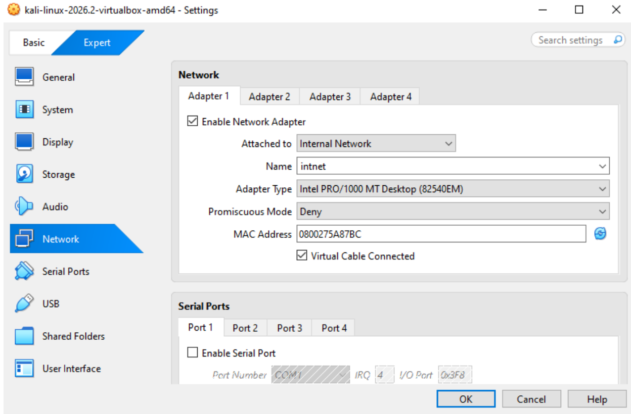
Figura 3. Configurarea la rețea „Internal Network”
